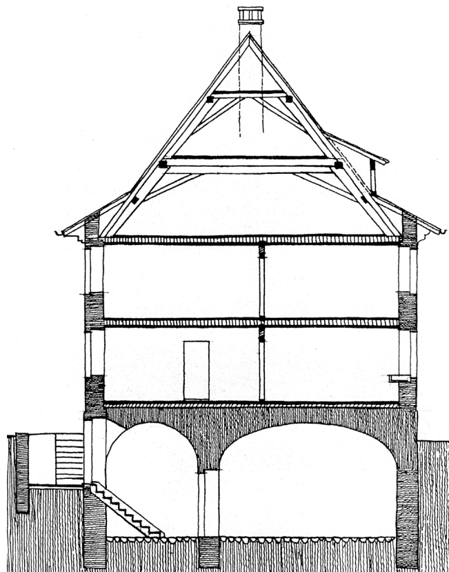
170. Rössligasse 44, Schnitt in einem Plan des Technischen Arbeitsdiensts Basel-Stadt von 1933.
