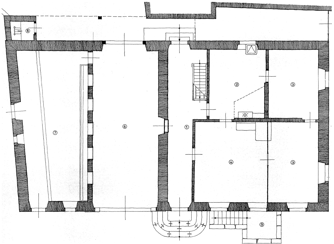
171. Rössligasse 44, Grundriss des Erdgeschosses in einem Plan des Technischen Arbeitsdiensts Basel-Stadt von 1933. 1 Gang; 2 Küche; 3 Zimmer; 4 Wohnzimmer; 5 Kellerabgang; 6 Scheune; 7 Stall; 8 Abort.
