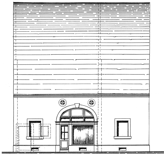
117. Baselstrasse 56, Strassenfassade im Plan für den Umbau von 1903. Links sind Tür und Fenster zum Stall gestrichelt angegeben.
