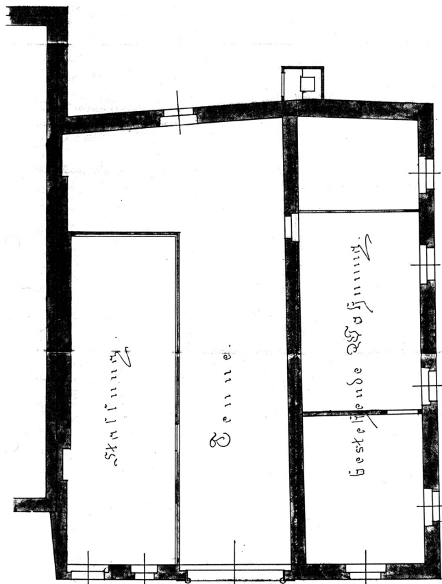
118. Baselstrasse 56, der Erdgeschossgrundriss vor dem Ausbau von Stall und Scheune (1903).
